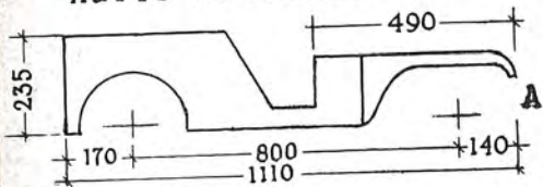
naris blatnika
