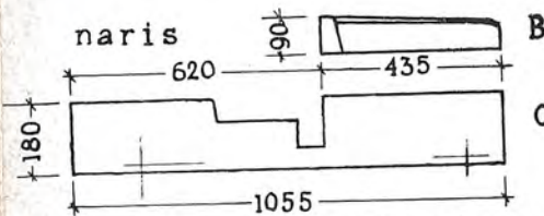
tloris sestavljenih delov ABC
