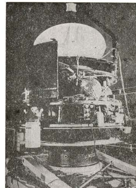
Vesoljska sonda »Giotto«, ki je priletela v neposredno bližino repatice in pošiljala na Zemljo izredne posnetke.
