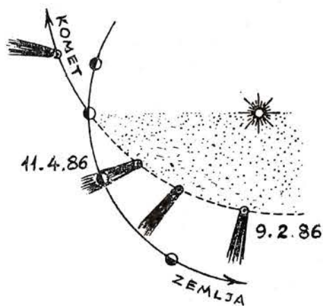
Zemlja in Halleyeva repatica si bosta najbližji 11. aprila 1986.
